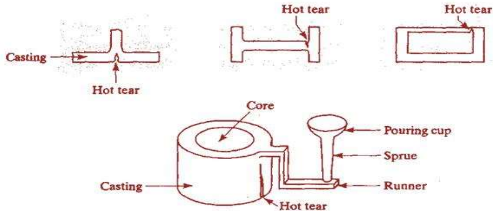
Fig Hot tears
